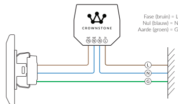
A) Inbouw Crownstone schakelschema. Pas op, de draadkleuren kunnen anders zijn.
