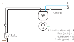
B) De Crownstone wordt geplaatst in het plafond.
